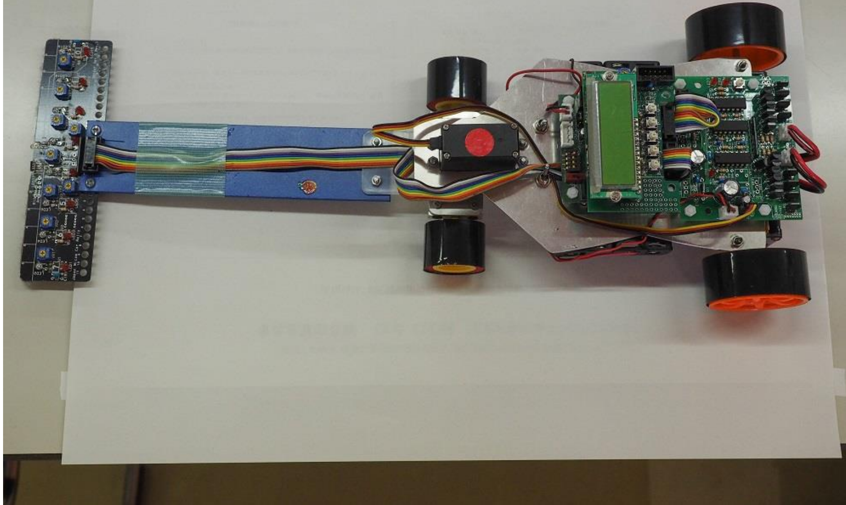
栃木県立那須清峰高等学校 小西 真気さん「清峰号」
